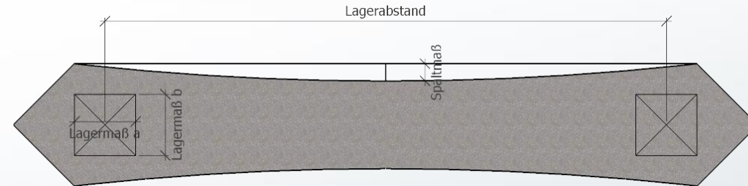
Das Spaltmaß des Kreissegmentes beträgt ca. 1/4 bis 1/5 des Lagermaßes b
